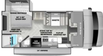
2251SLE (Available on Ford E350/Chevy 3500)
