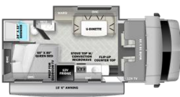
2151SLE (Available on Ford E350/Chevy 3500)
